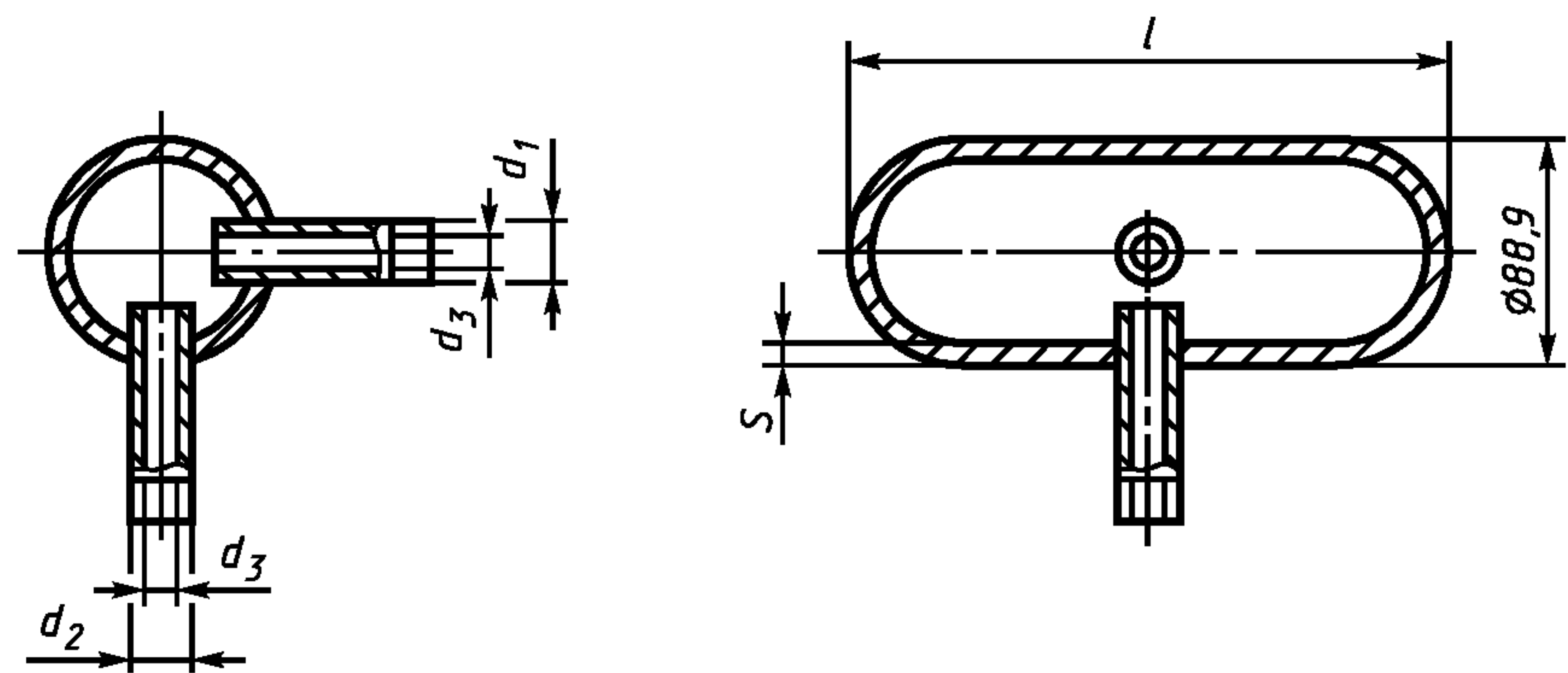
Рисунок 1 — Уравнительные сосуды
