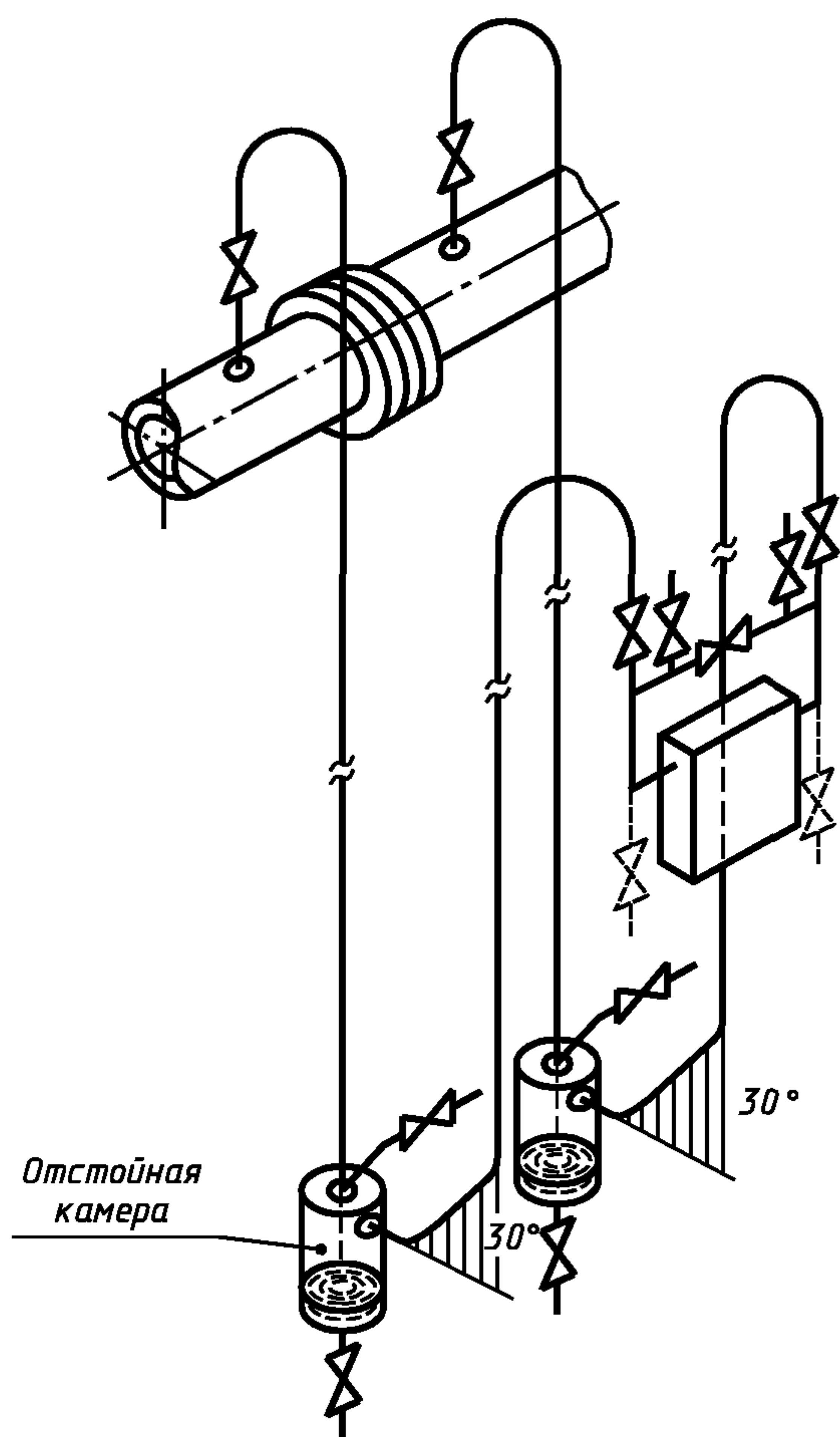
Рисунок Г.9 — ППД под трубопроводом
