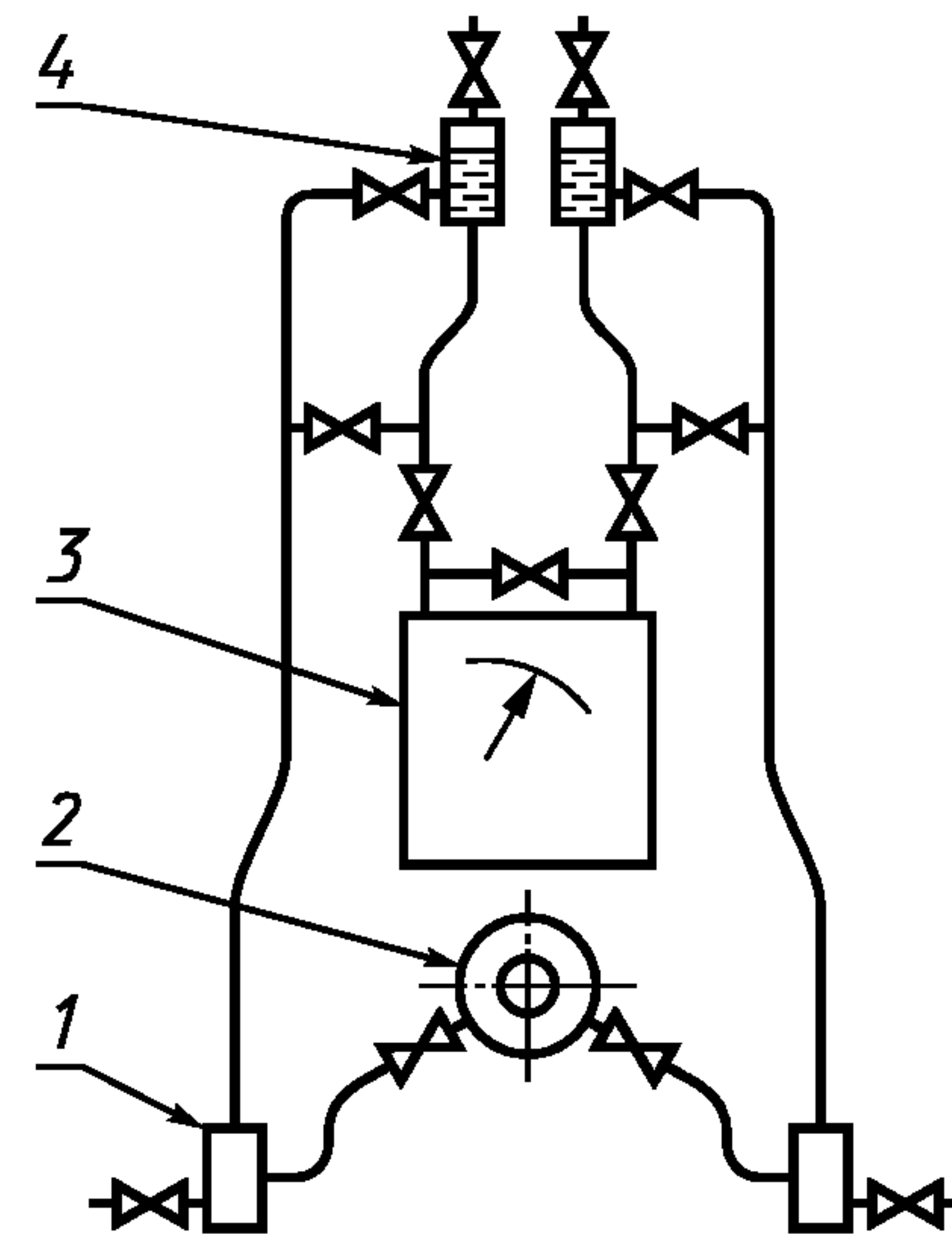
1 — отстойная камера; 2 — СУ; 3 — ППД; 4 — воздушосборник
