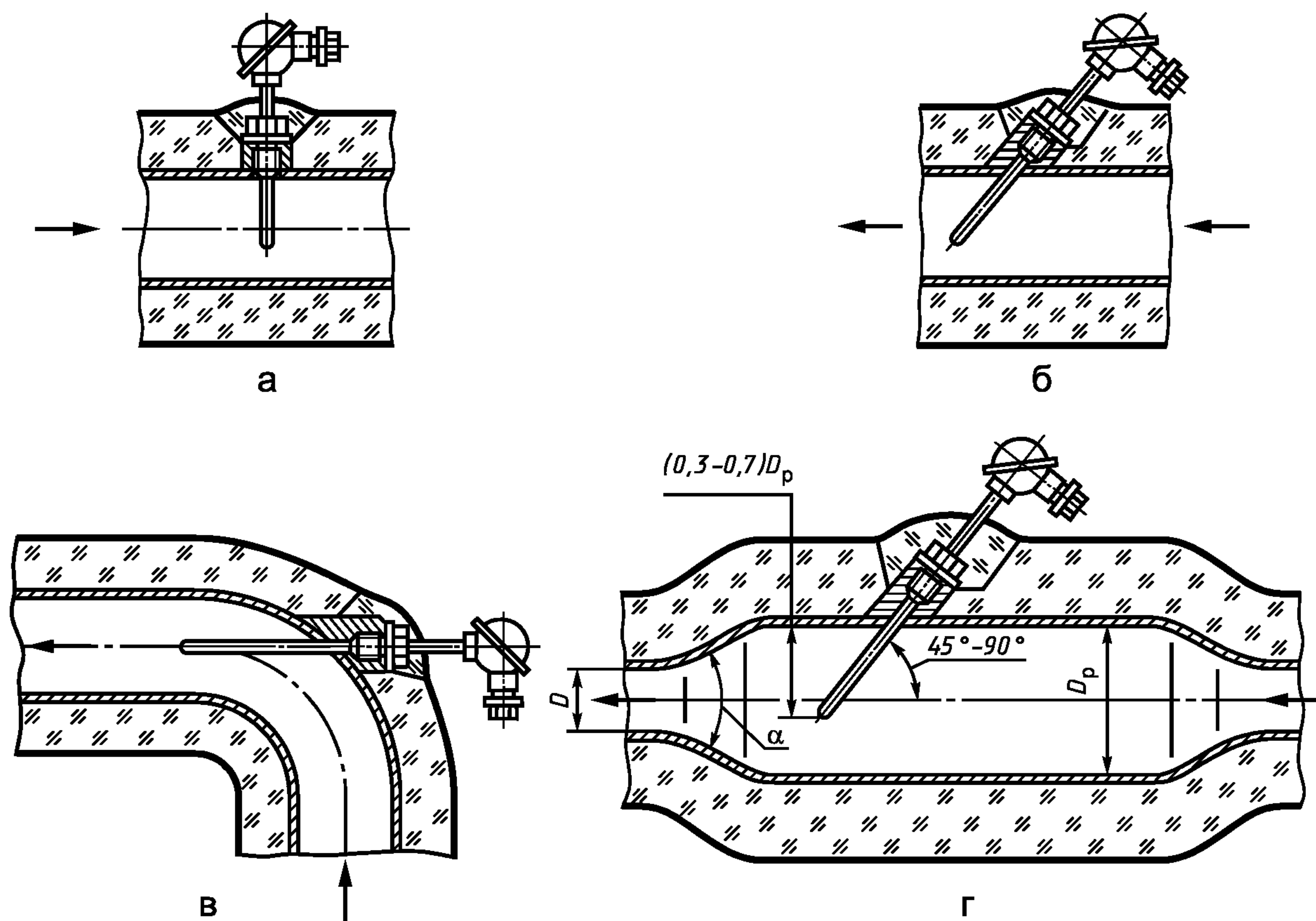
Рисунок 11 — Схема установки ПТ
