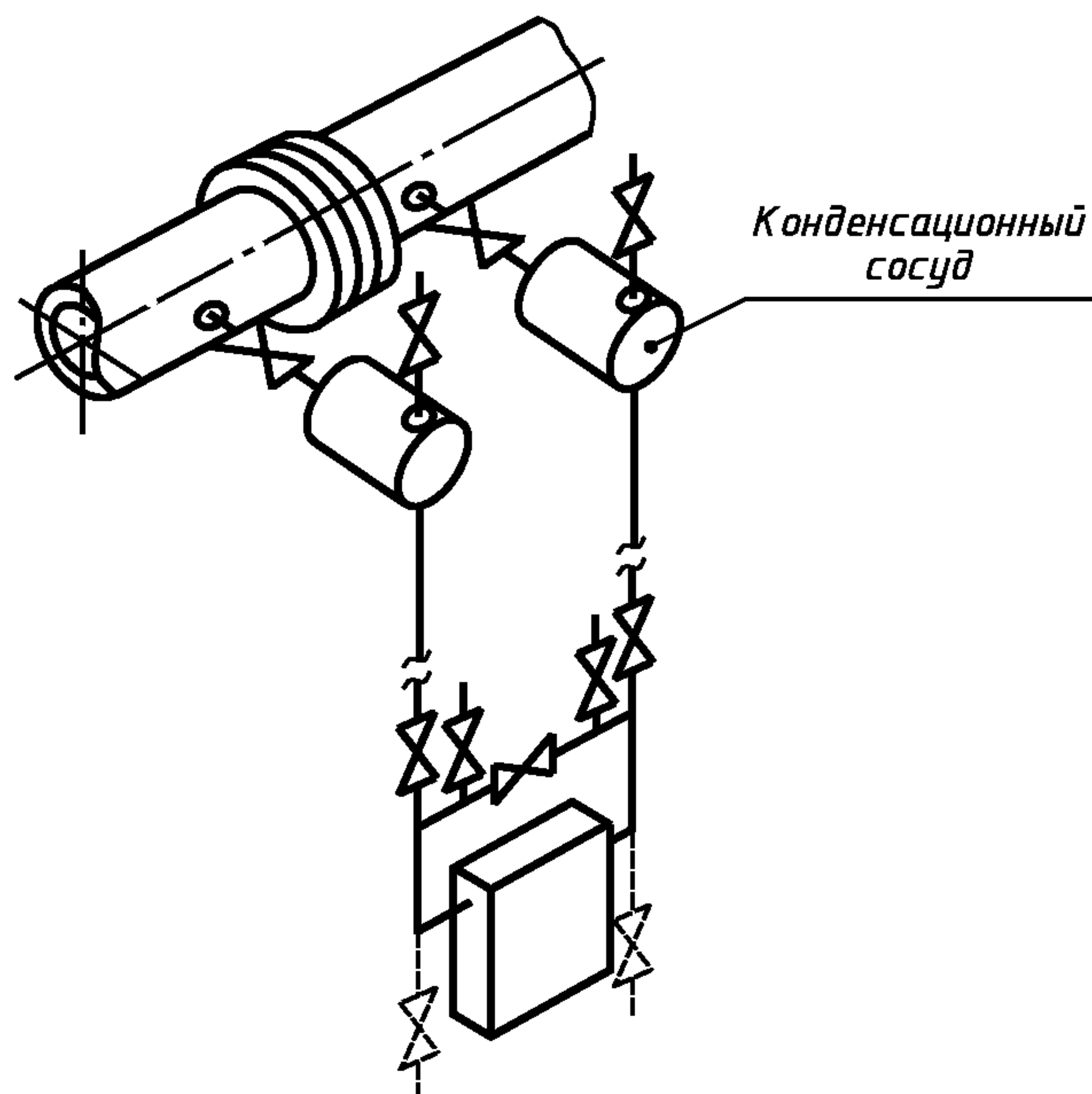
Рисунок Г.5 — ППД под трубопроводом
