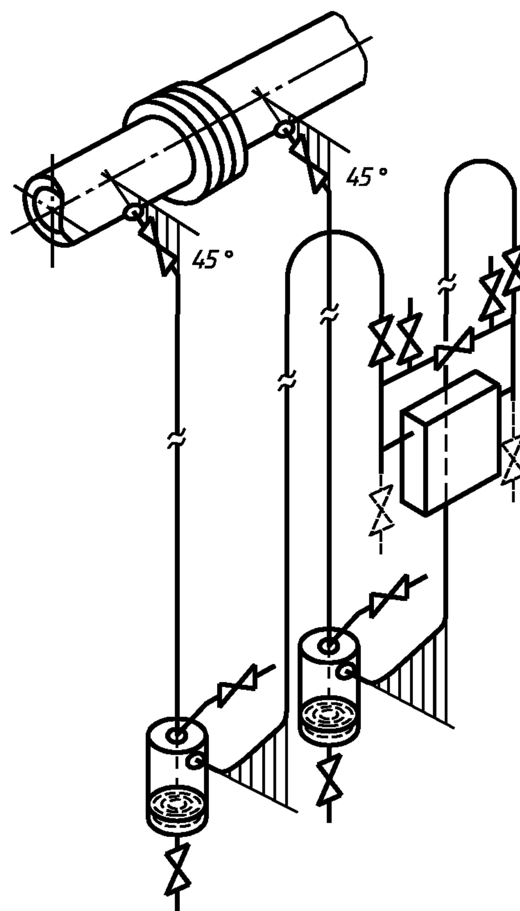
Рисунок Г.10 — ППД под трубопроводом (вариант)
