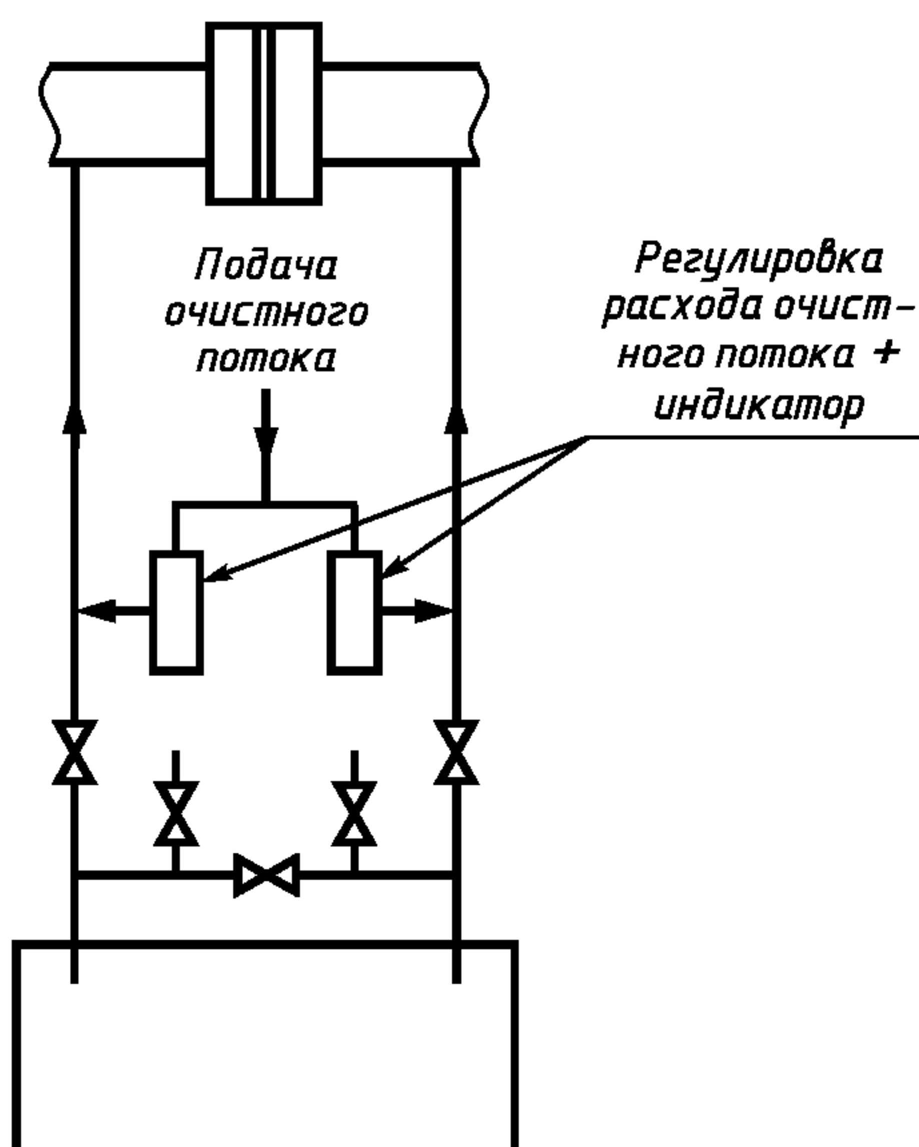
Рисунок 9 — Пример установки очистной системы
