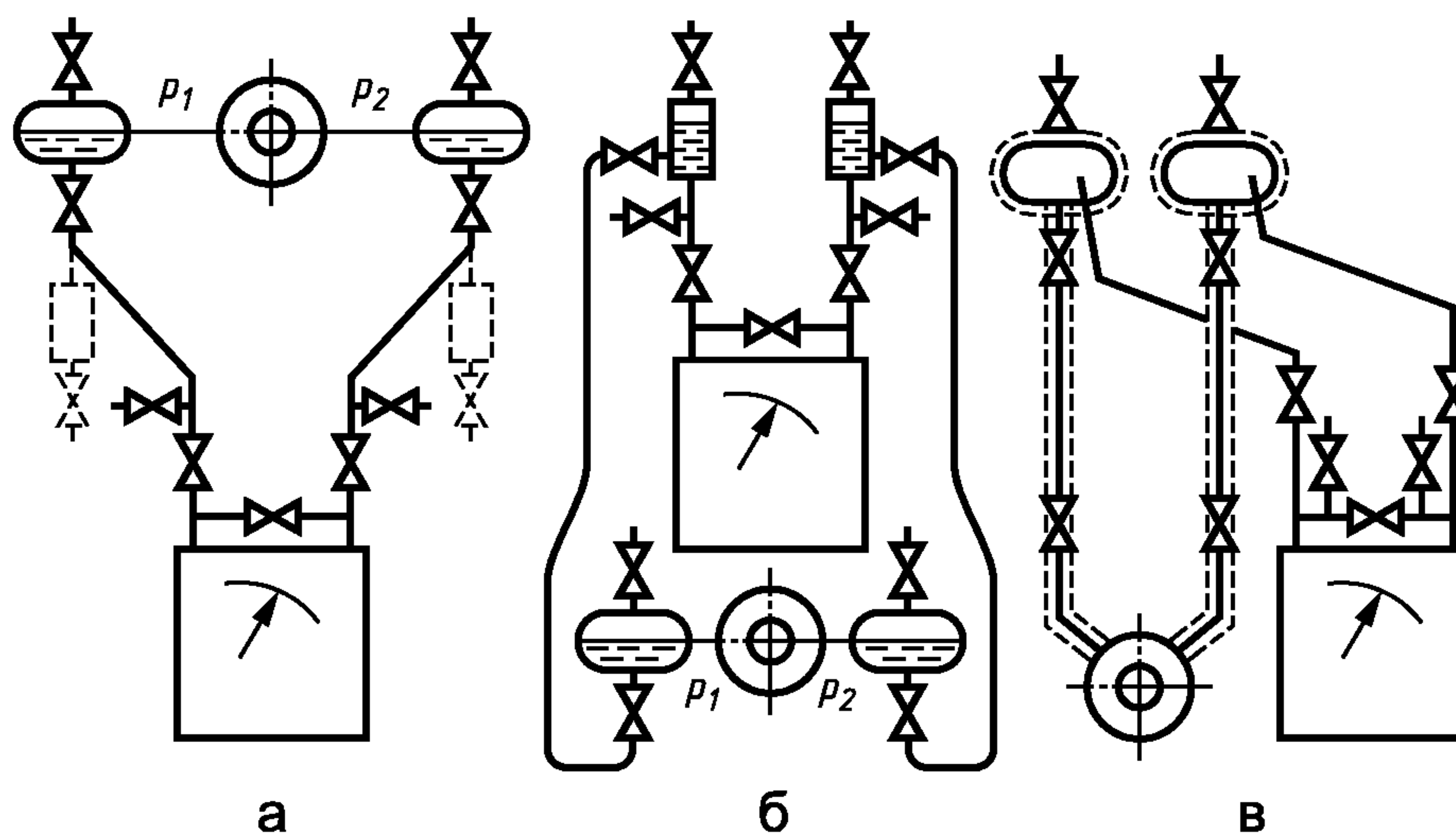
Рисунок 3 — Схемы расположения уравнильных сосудов и соединительных трубок
