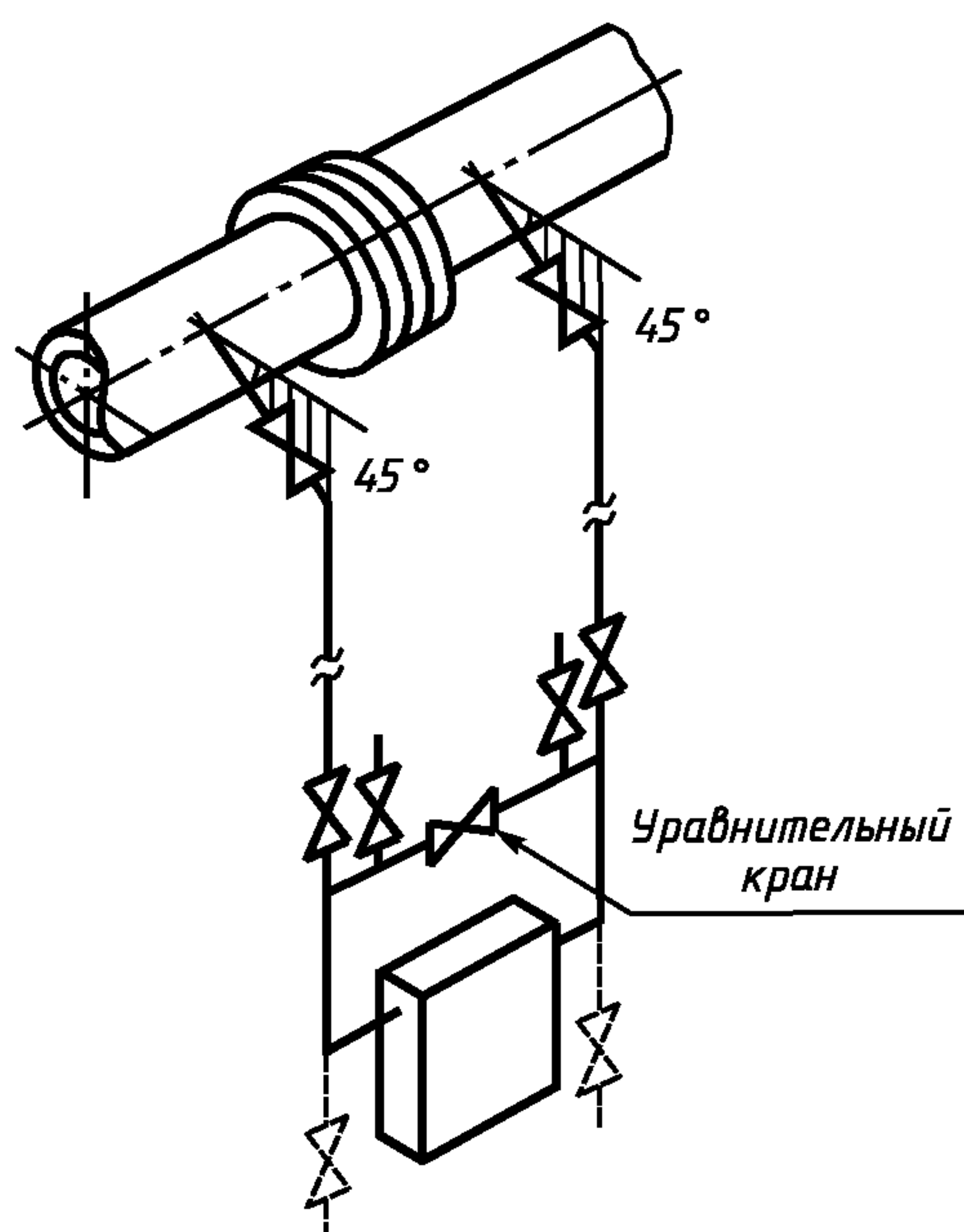
Рисунок Г.15 — ППД под трубопроводом
