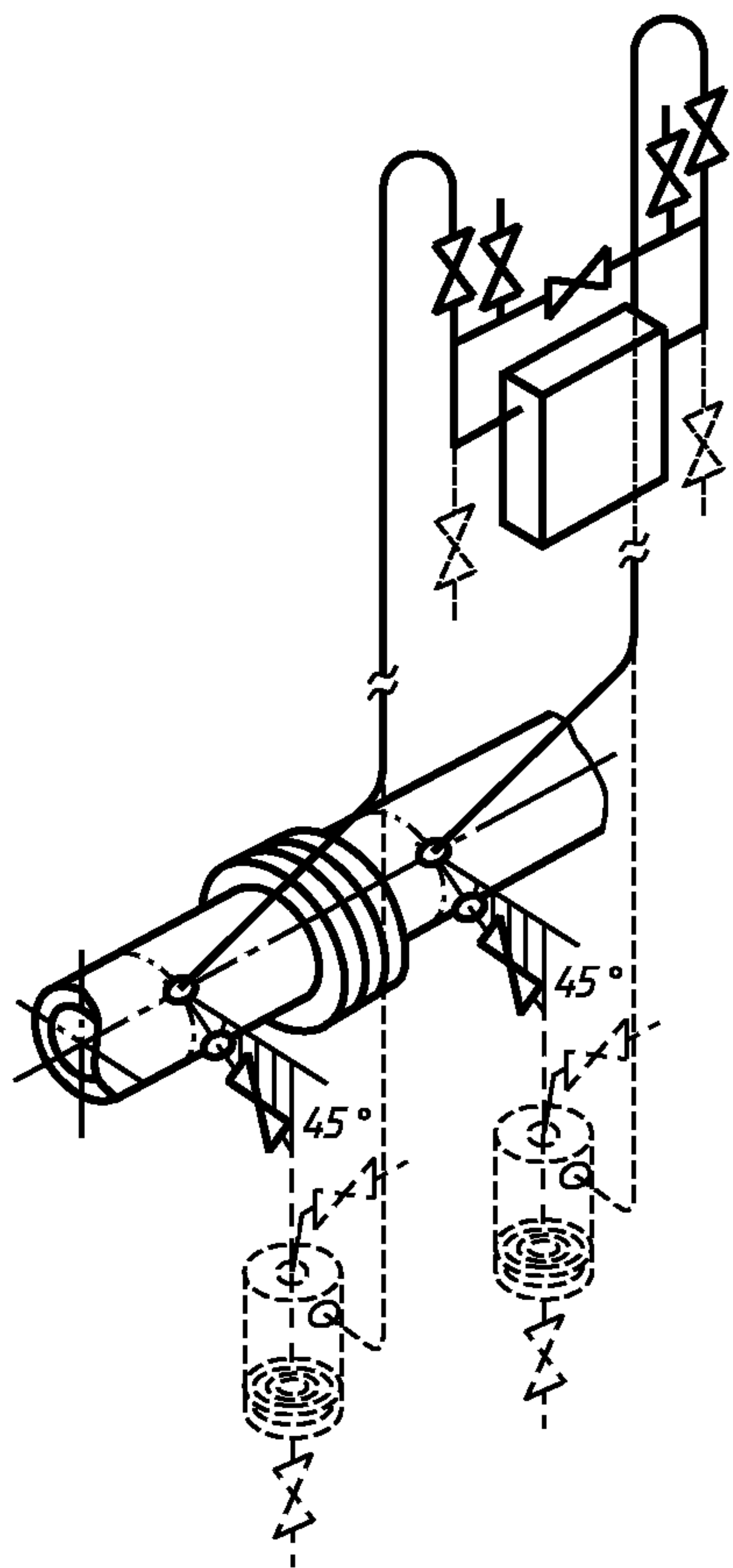
Рисунок Г.11 — ППД над трубопроводом (два варианта)
