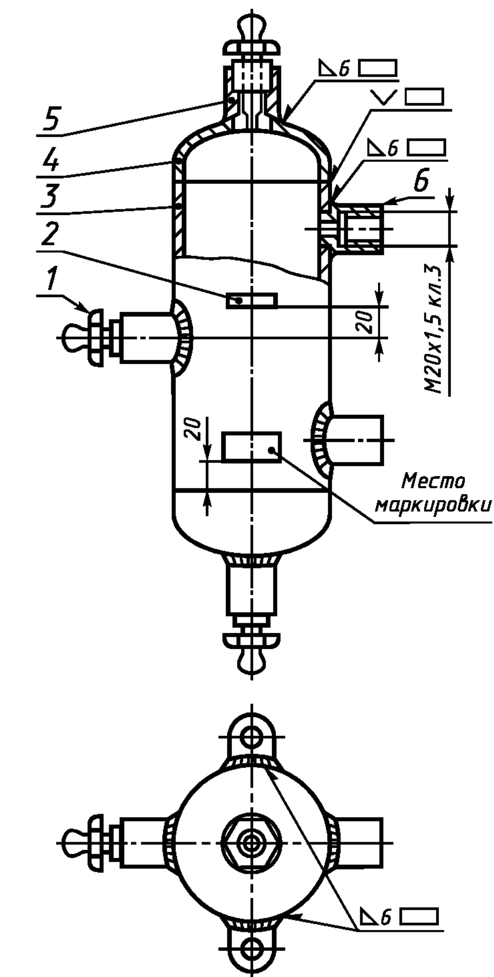
1 — пробка; 2 — ушко; 3 — обечайка; 4 — днище; 5 — штуцер; 6 — штуцер
