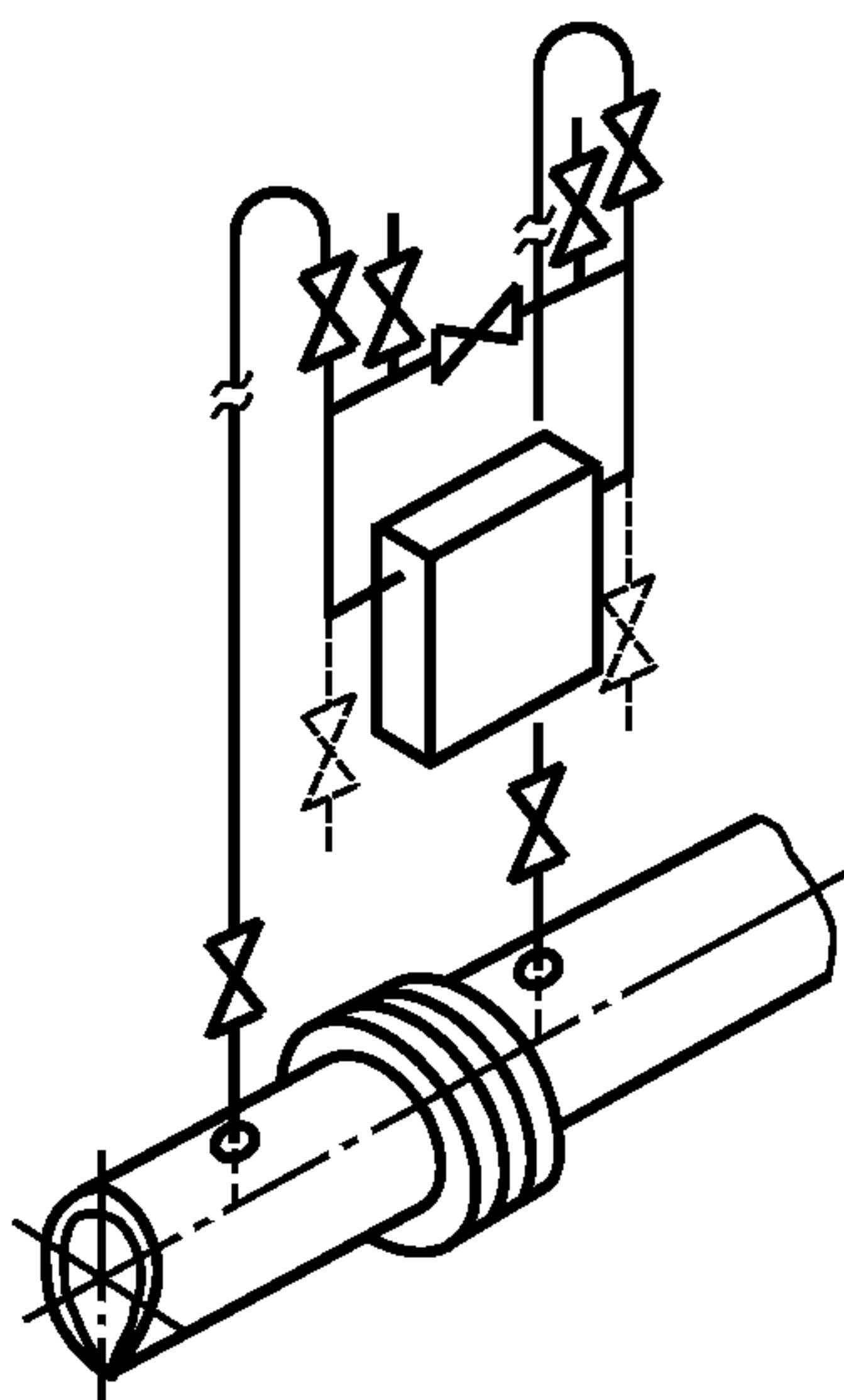
Рисунок Г.1 — ППД над трубопроводом
