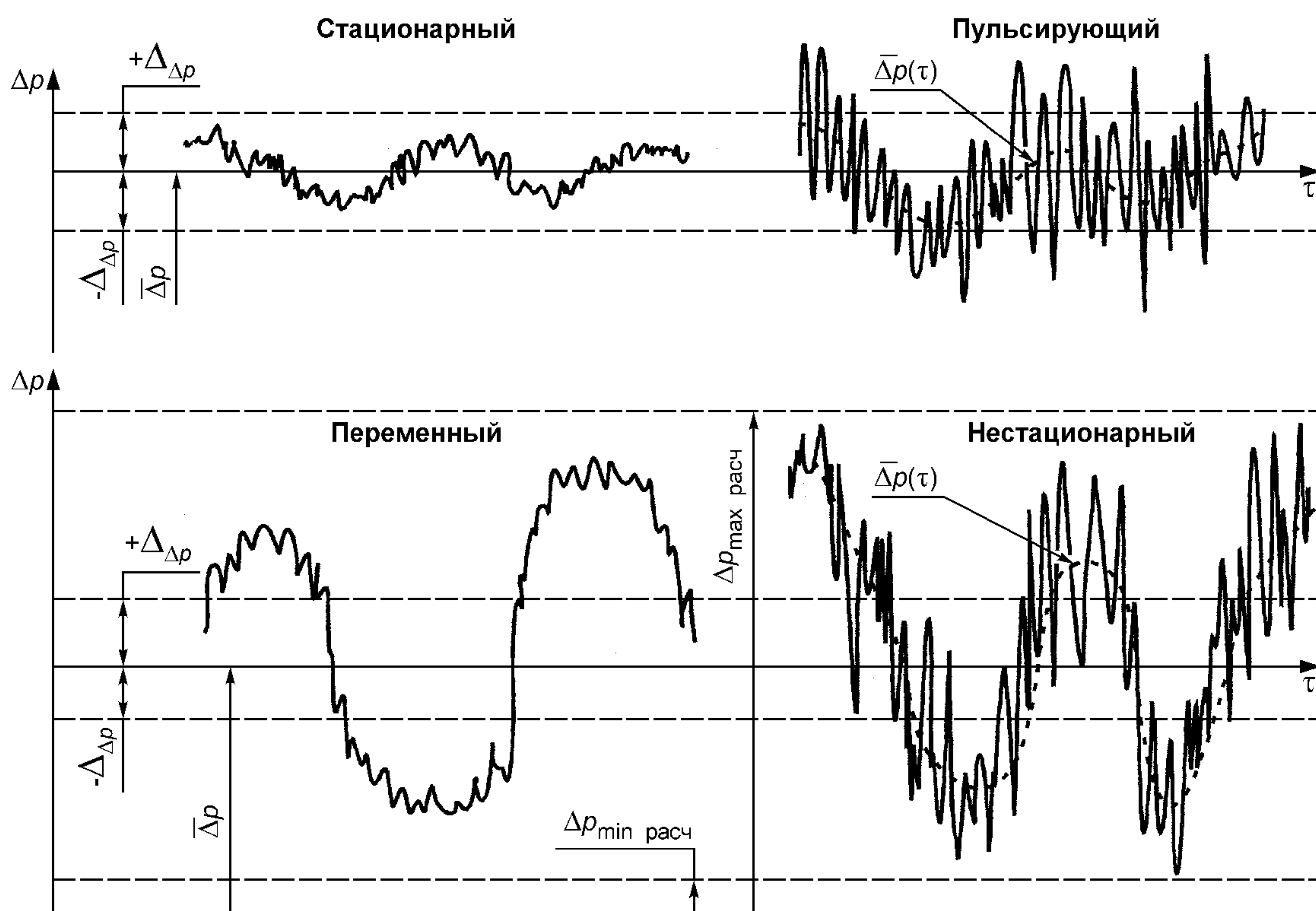
Рисунок Ж.2 — Характер изменения \Delta p(\tau)
