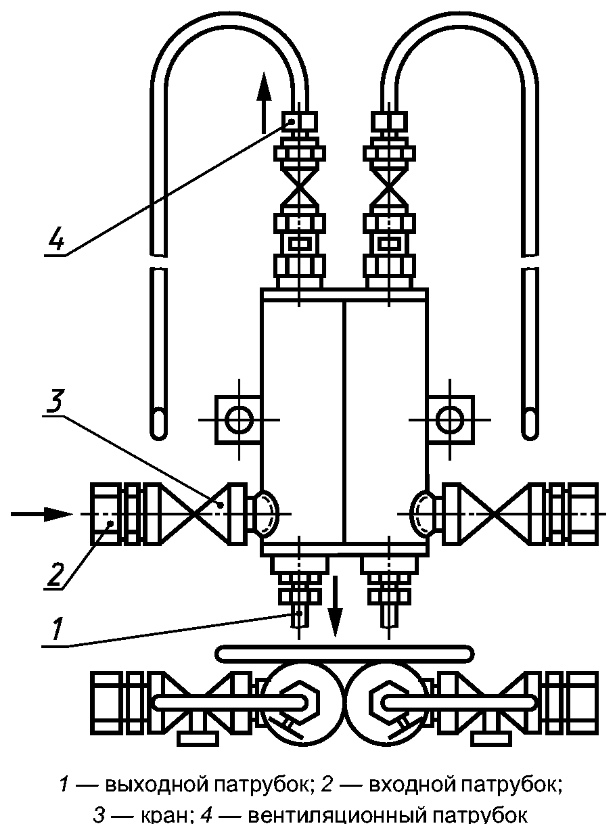
Рисунок 7 — Газосборные камеры
