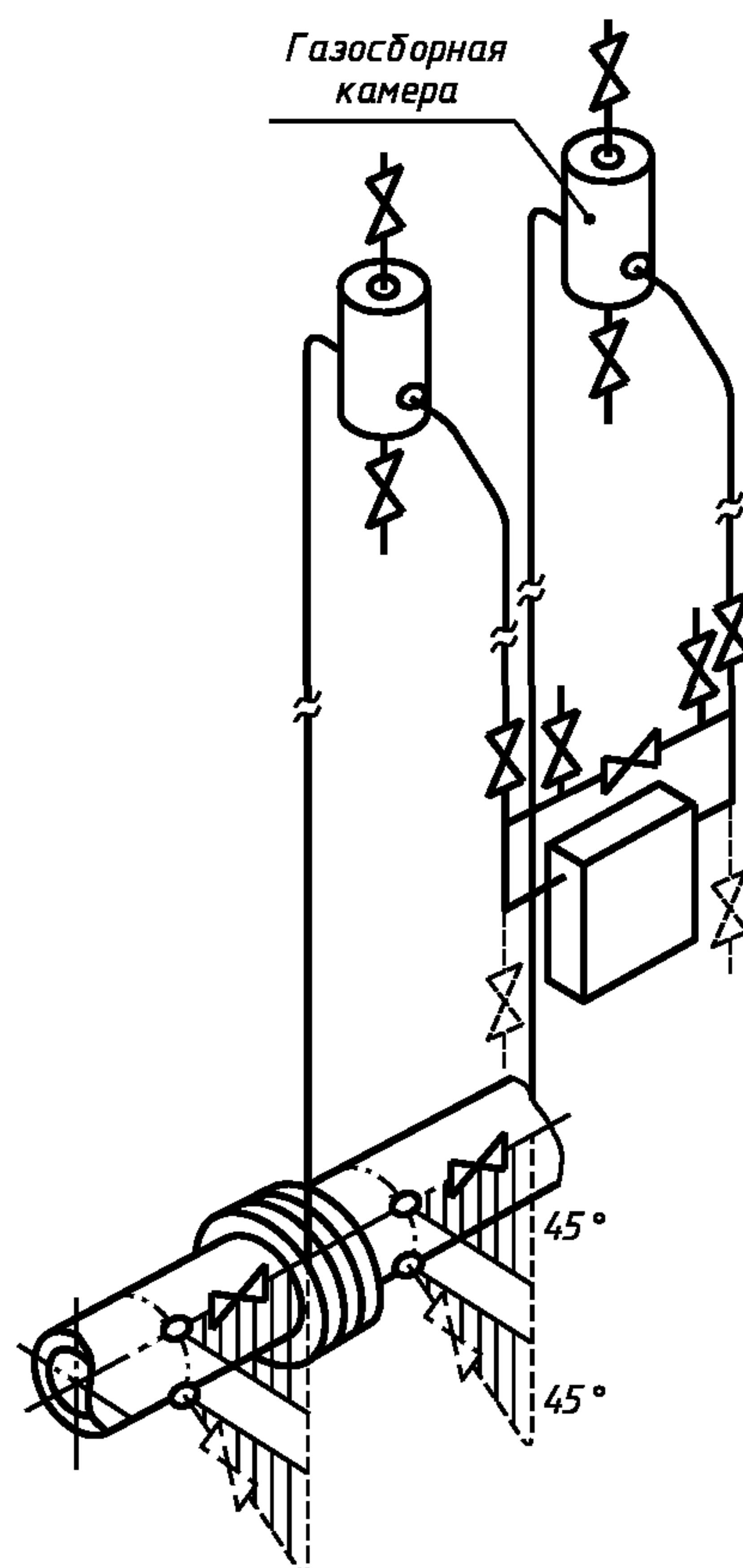
Рисунок Г.16 — ППД над трубопроводом
