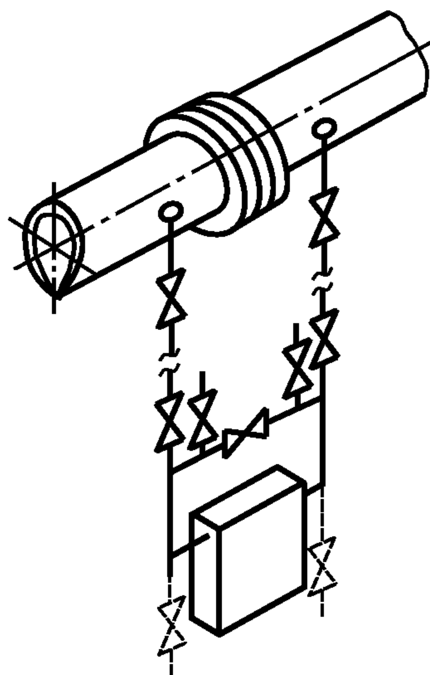
Рисунок Г.2 — ППД под трубопроводом
