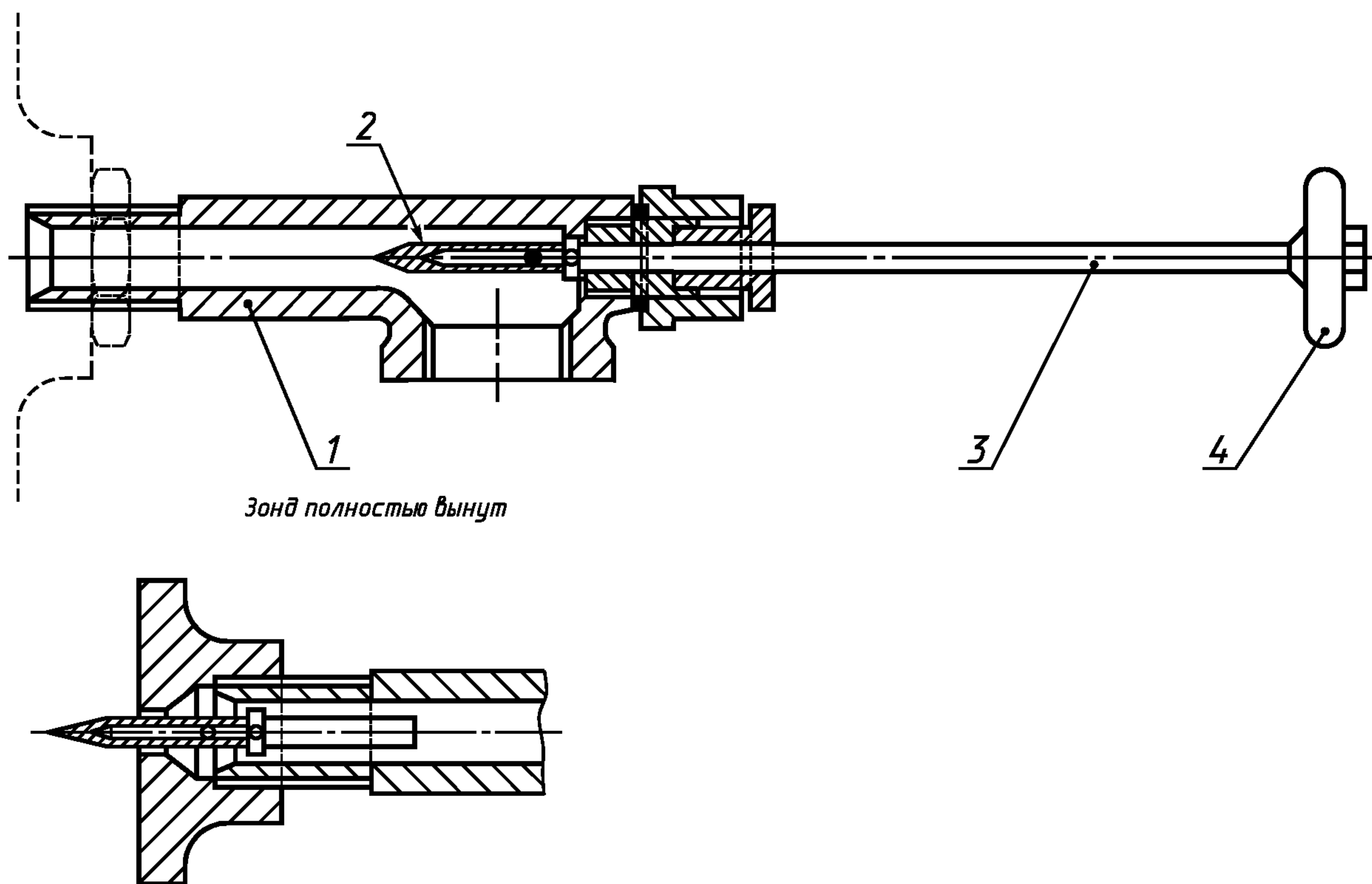
1 — корпус; 2 — головка зонда; 3 — ось зонда; 4 — рукоятка
