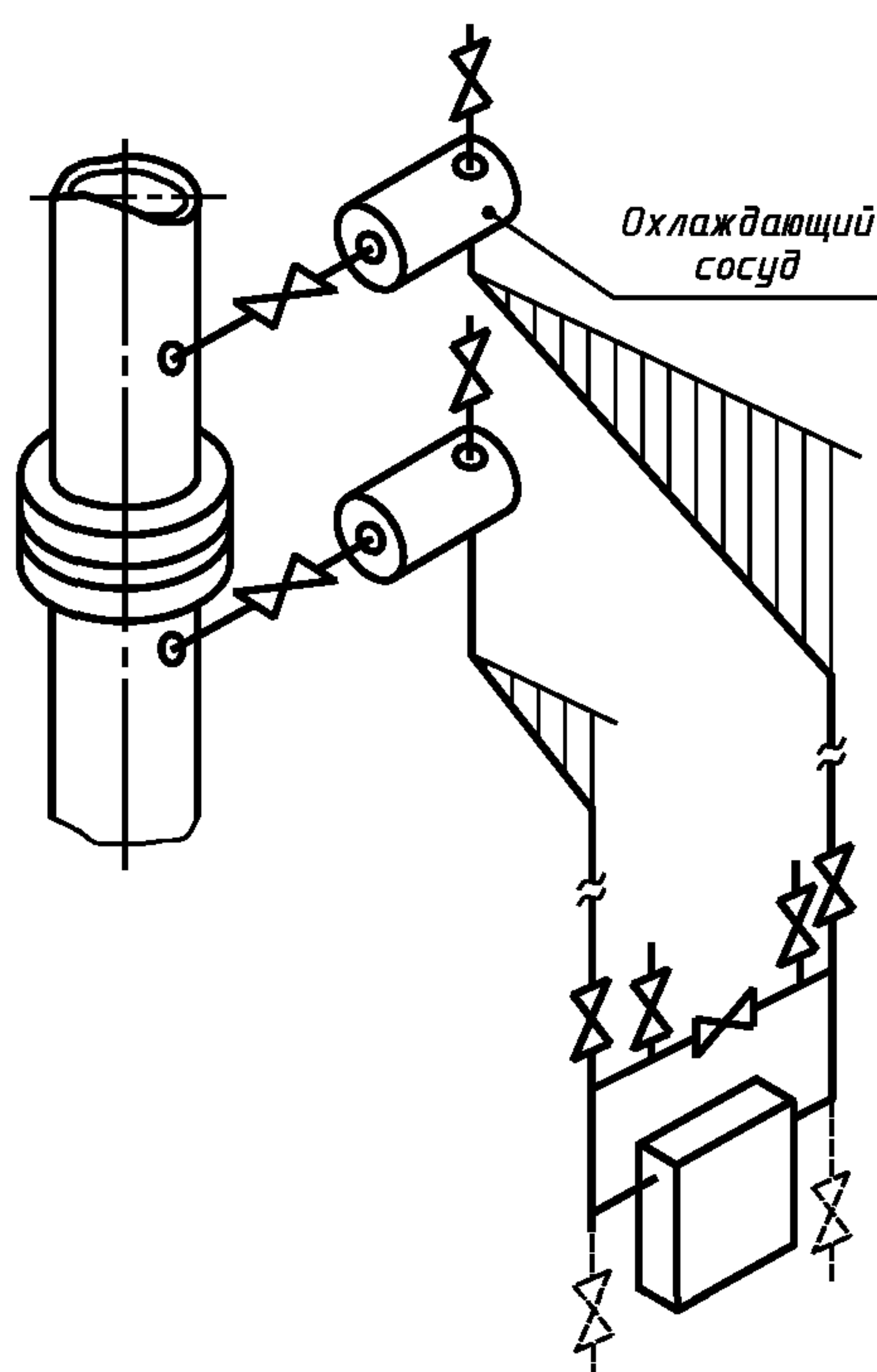
Рисунок Г.17 — Вертикальный трубопровод
