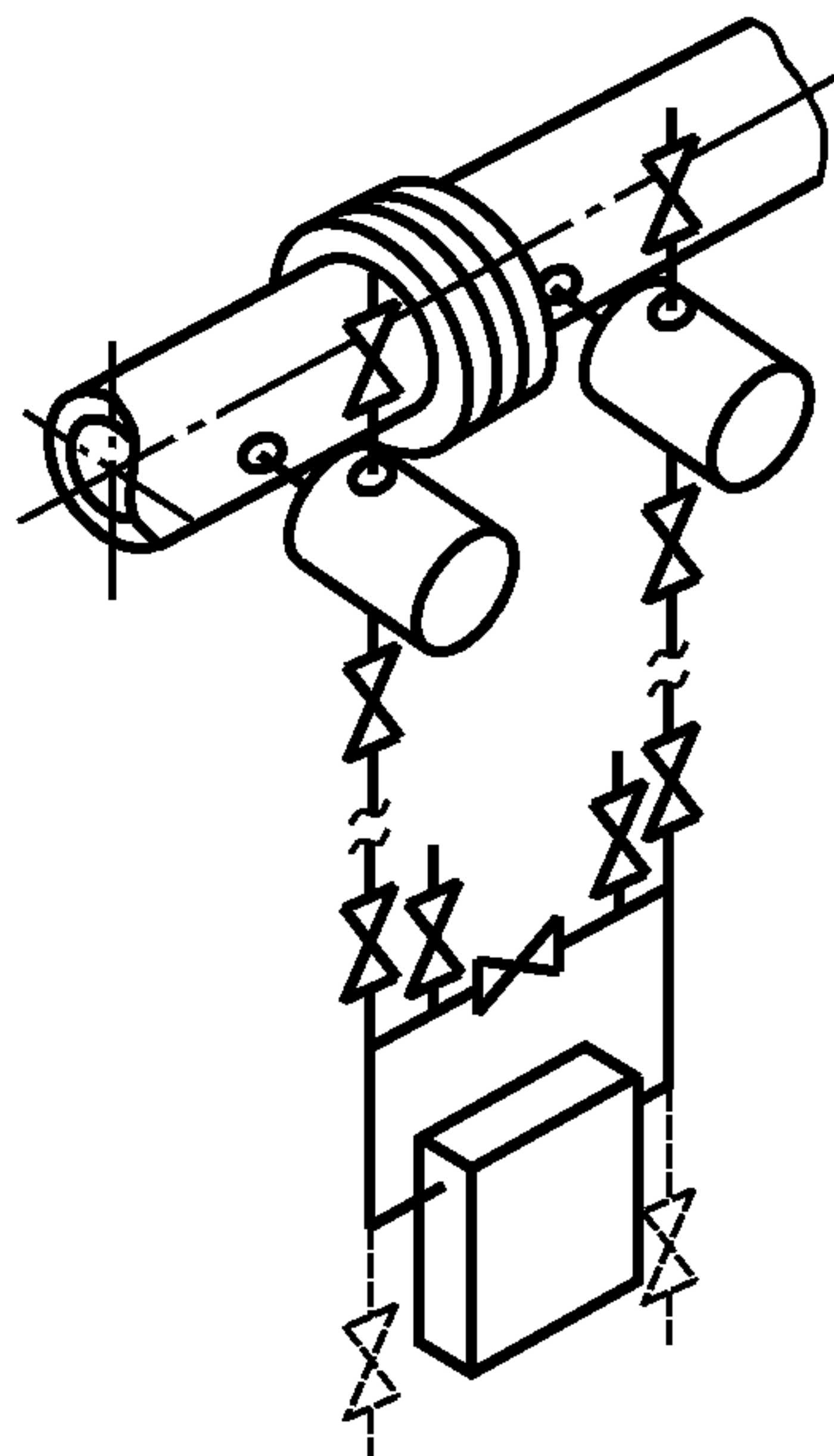
Рисунок Г.6 — ППД под трубопроводом (вариант)
