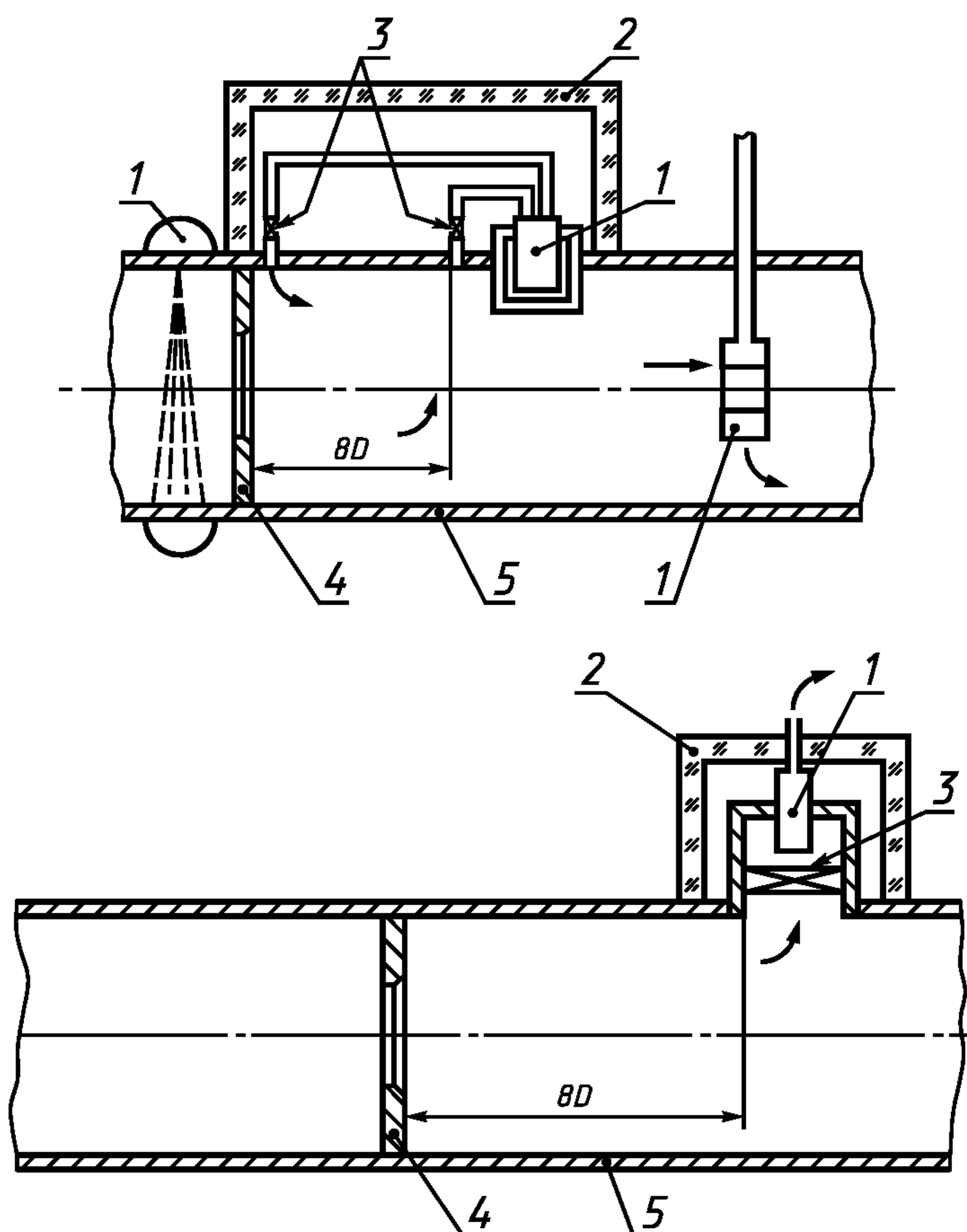
1 — плотномер; 2 — теплоизоляция; 3 — вентиль; 4 — сужающее устройство; 5 — трубопровод
